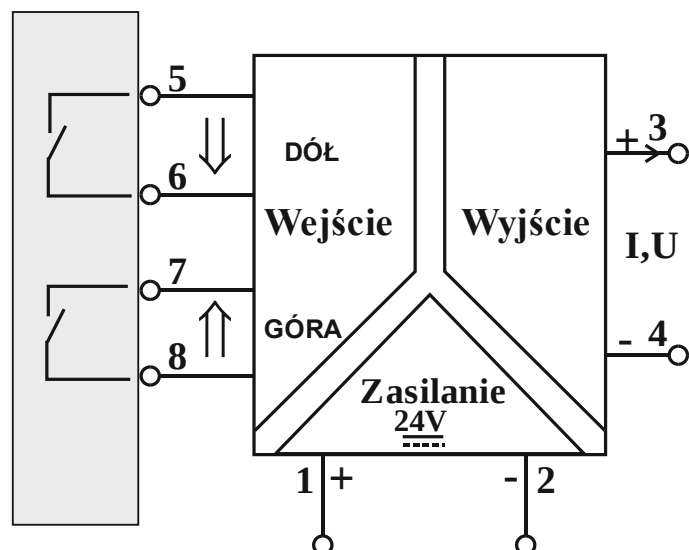
Rys.2 Schemat funkcjonalny przetwornika ZIU-S2. Sposób podłączania sygnałów binarnych
