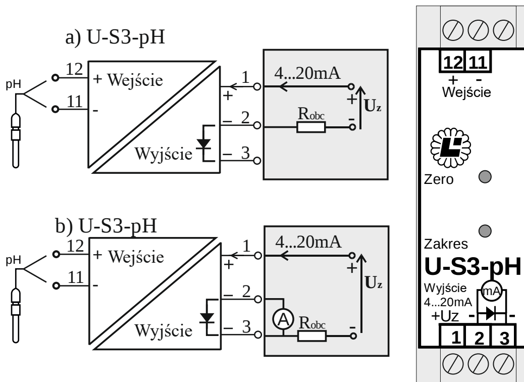
Rys.2 Schemat blokowy oraz opis zacisków podłączeniowych przetwornika U-S3-pH
