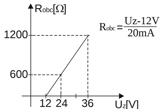
Rys.1 Sposób wyznaczenia rezystancji obciążenia
