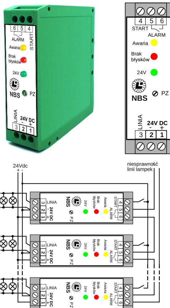
Rys. 1 Schemat podłączeniowy przy kilku liniach lamp błyskowych
