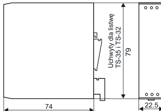
Rys. 2 Wymiary obudowy
