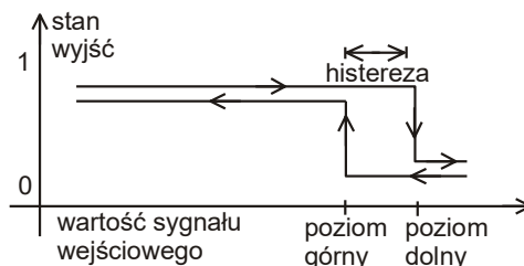
Rys.2 Przebieg stanu wyjść dla alarmu MINIMUM
