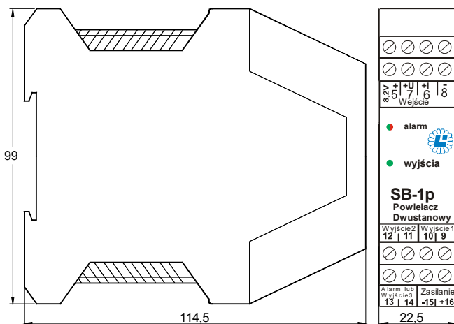
Rys.1 Szkic obudowy. Widok strony czołowej
