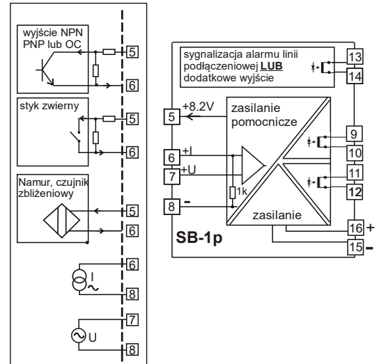
Rys.2 Opis zacisków podłączeniowych separatora SB-1p.
