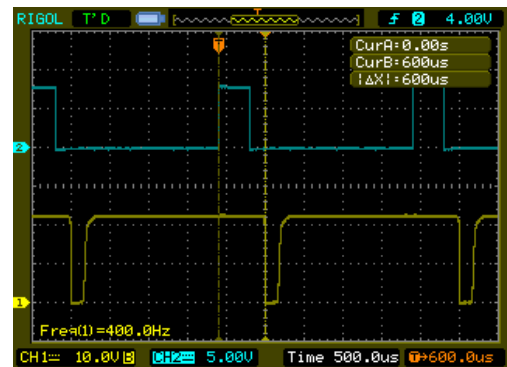
Rys. 3 Odpowiedź wyjścia OPTO.
